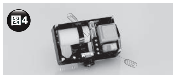
第2、3颗螺丝接电源线
