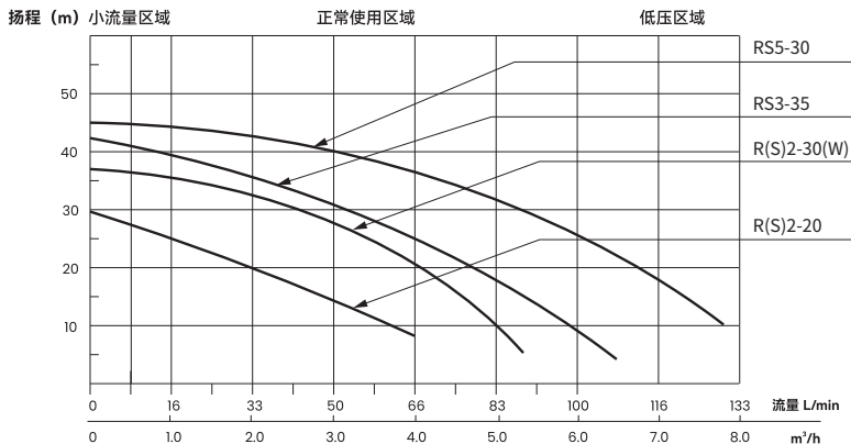
永磁变频增压泵R系列性能曲线图
