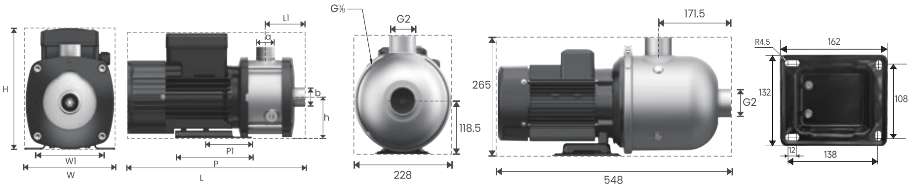
产品安装尺寸:
