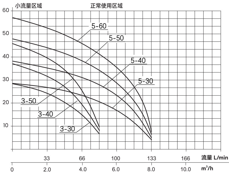
不锈钢多级离心泵性能曲线图
