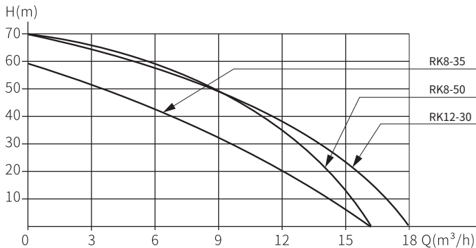
永磁变频多级离心泵RK系列性能曲线图
